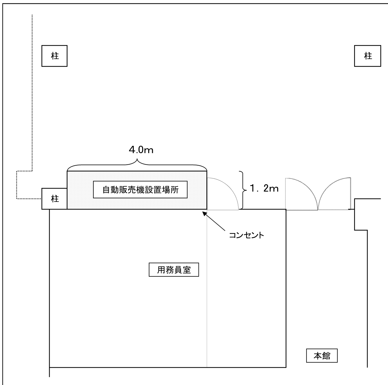
設置場所見取り図
